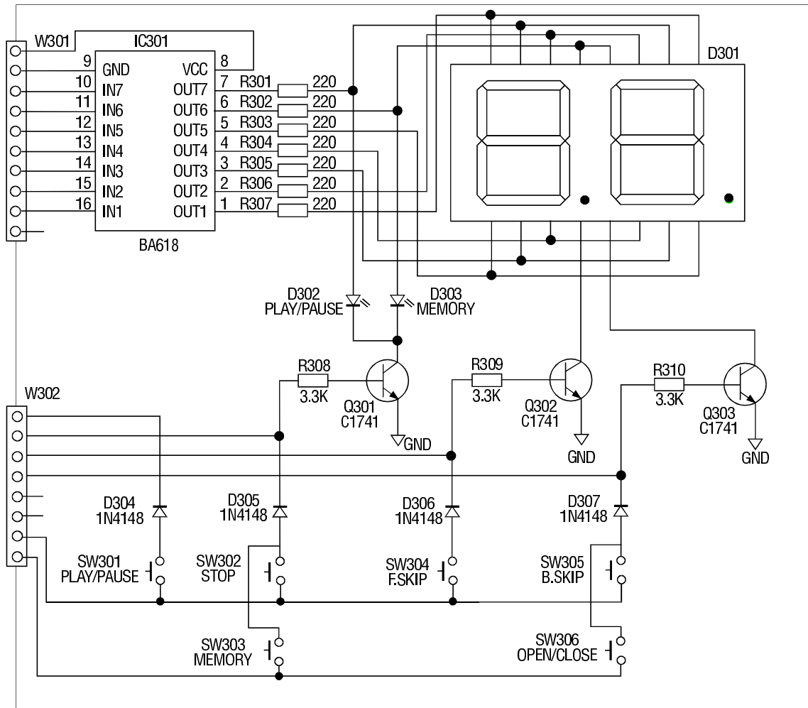
MODEL KE-400
